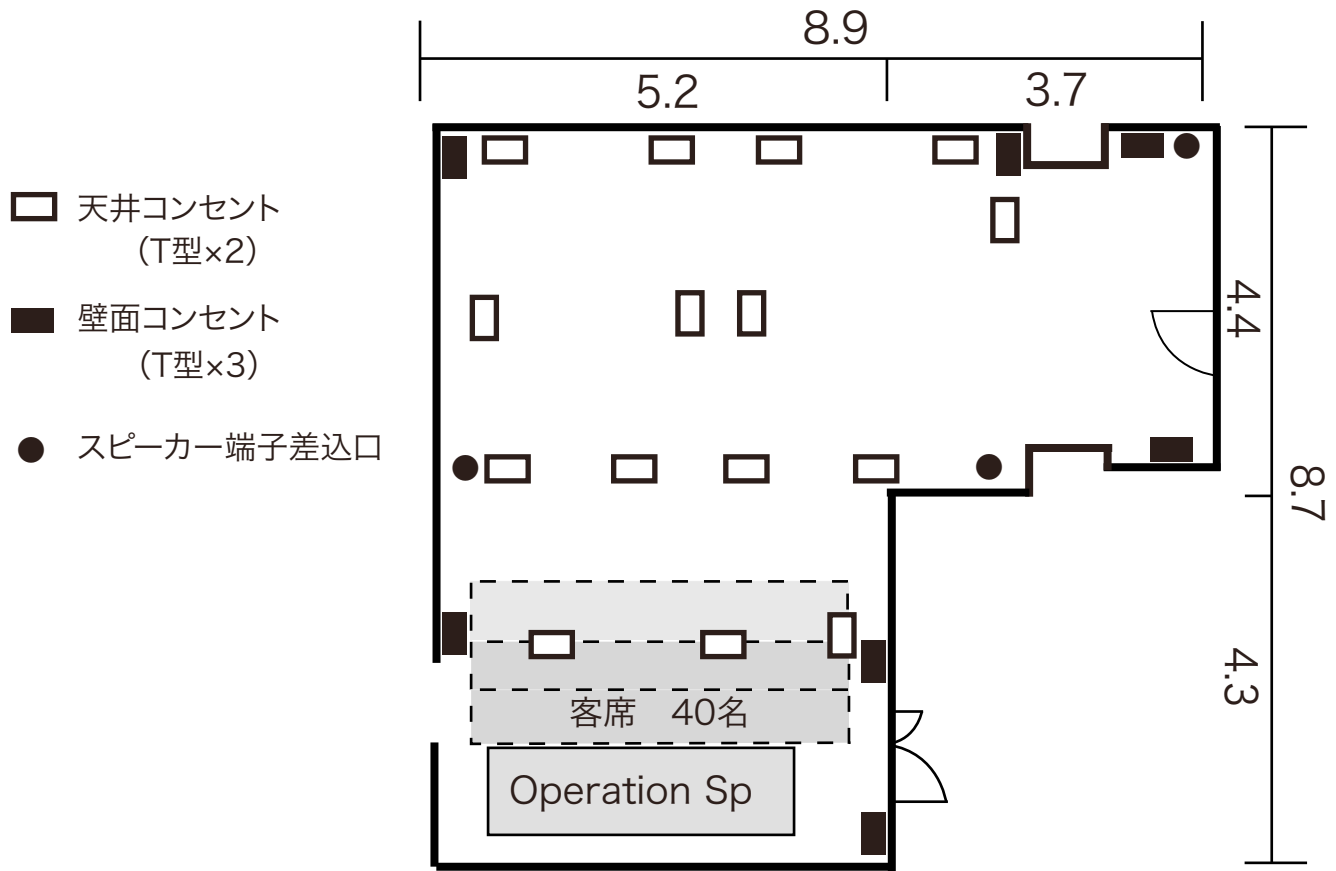
-配電図-
