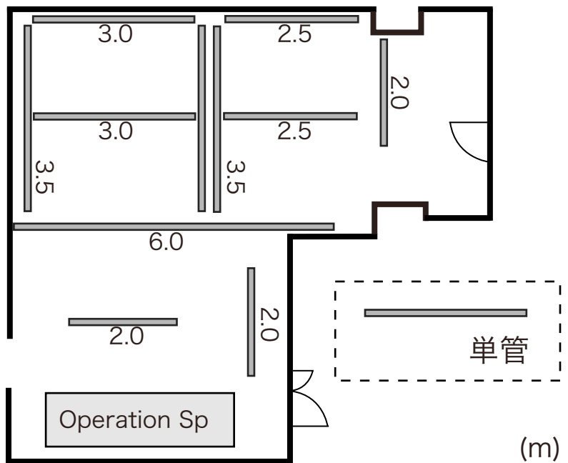
-灯体取り付け用単管配置図-
